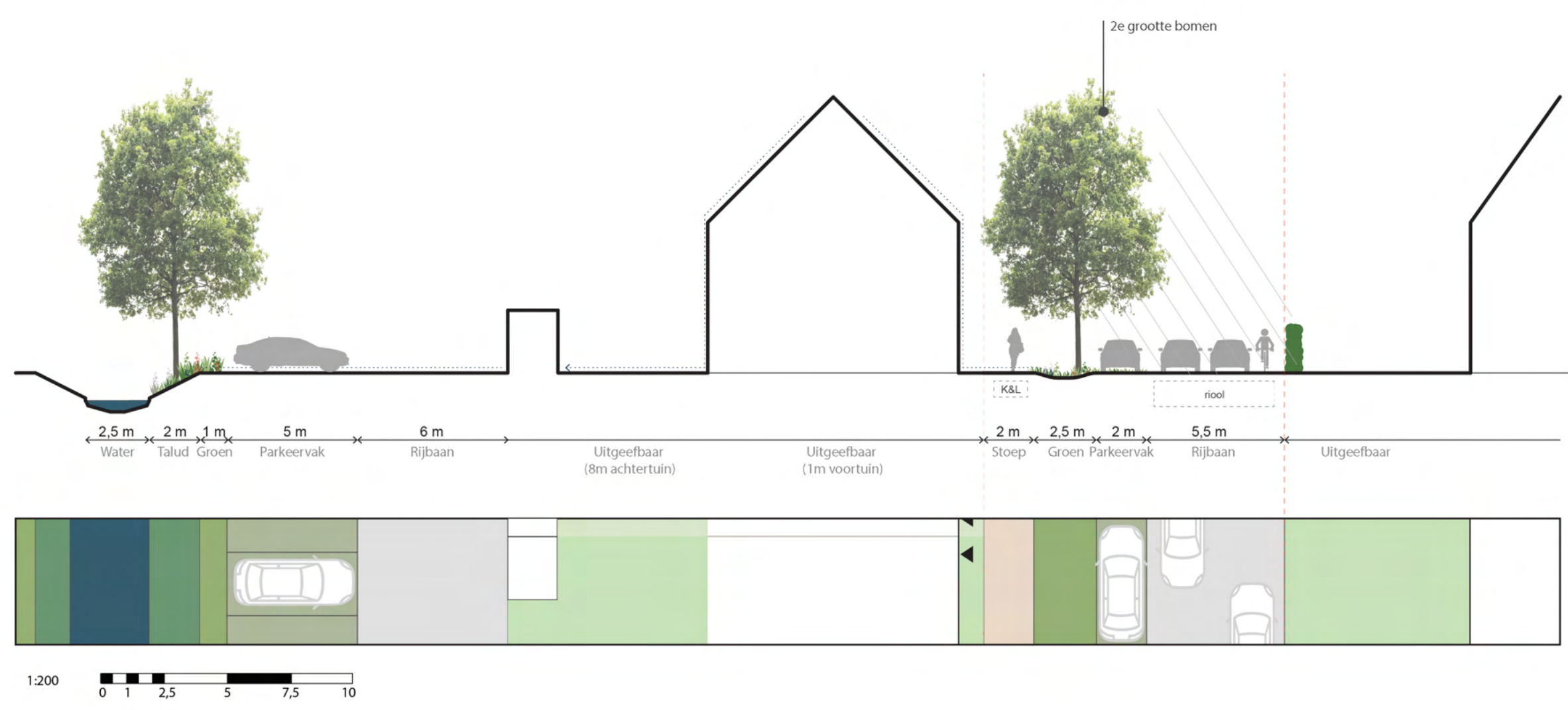
Profiel C - woonstraat
