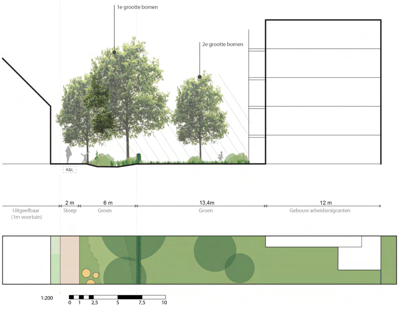
Profiel B - noordzone langs het groen
