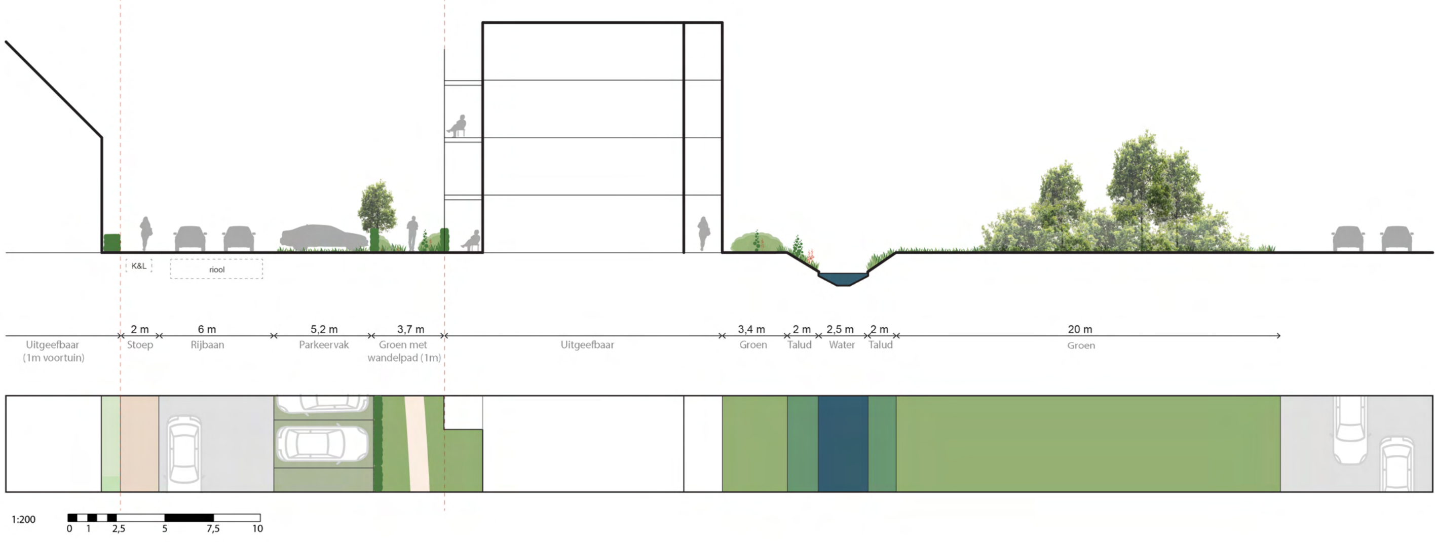
Profiel D - noordzone
